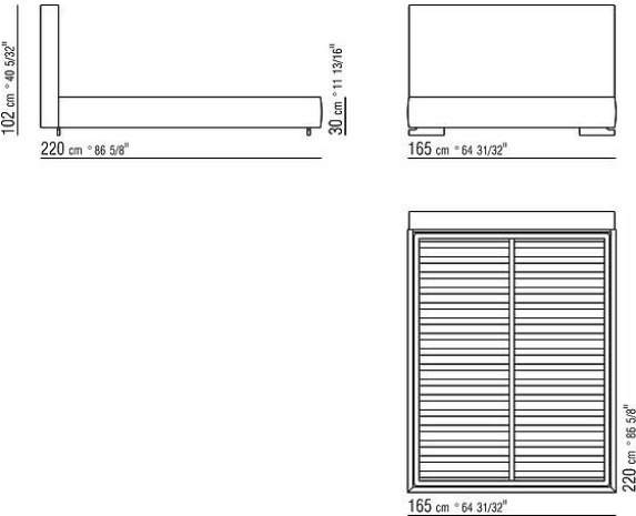
COD. 011UM1 BED W/ SLATS
