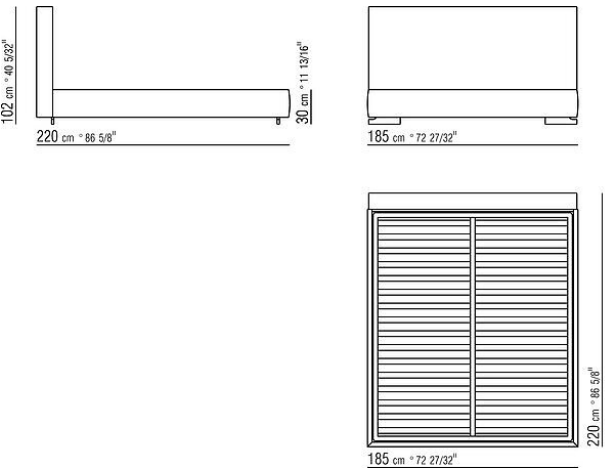
COD. 011UM3 BED W/WOODEN SLATS
