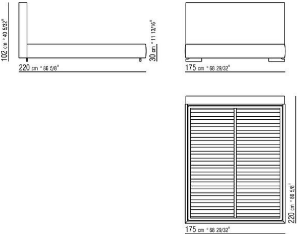
COD. 011UM2 BED W/ SLATS
